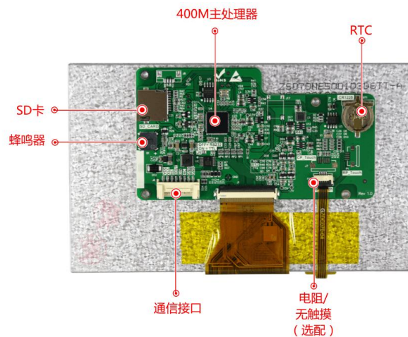
图 1-3 硬件配置图
